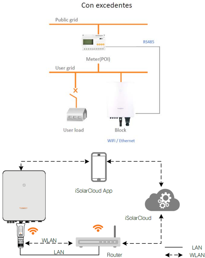
Imatge 6. Esquema Monitorització
