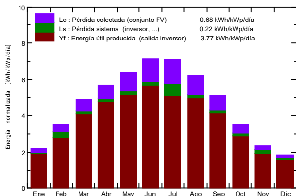
Producciones normalizadas (por kWp instalado): Potencia nominal 13.20 kWp
